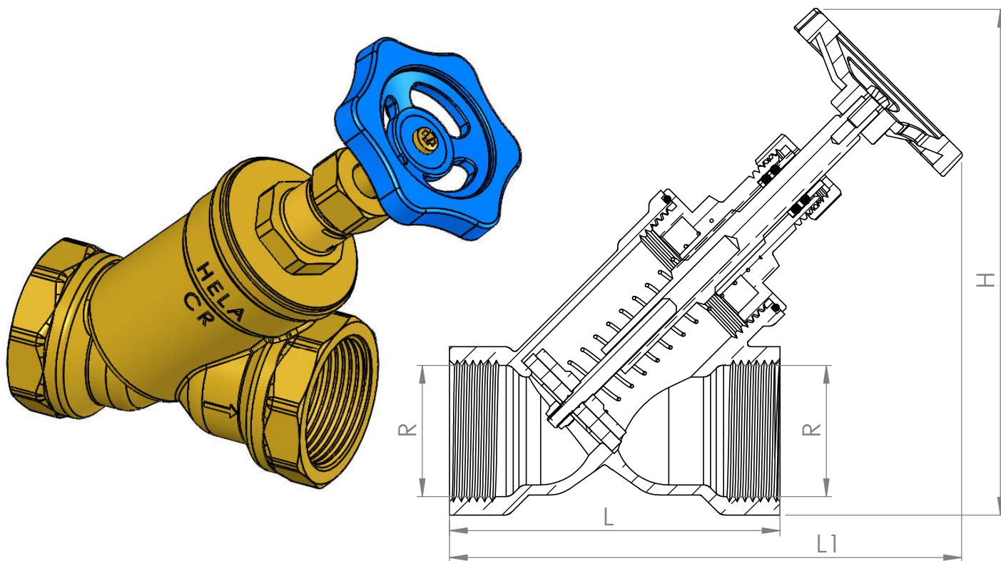
342 Takaiskuventtiili sululla
